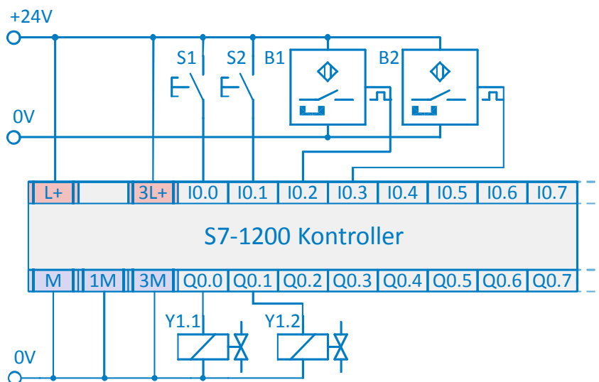
Elektriskeem
