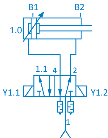
Pneumoskeem
