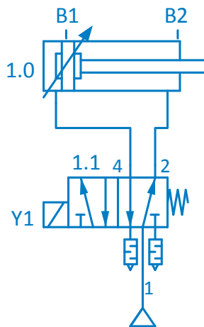
Pneumoskeem
